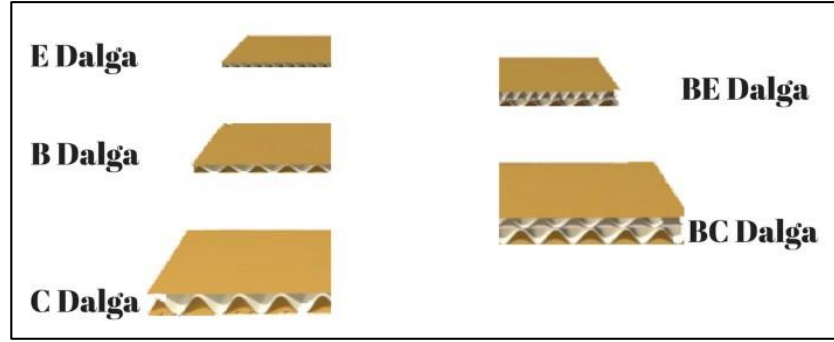
Görsel 2.13. Oluklu Mukavvaların Dalga Tipleri (Kâğıt Boyutu, 2018)
